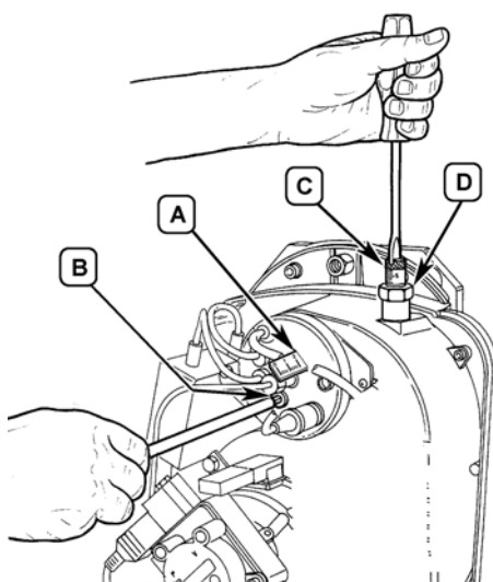
fig. 26 - Regolazione bruciatore
