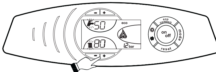
fig. 23 - Modalità TEST
