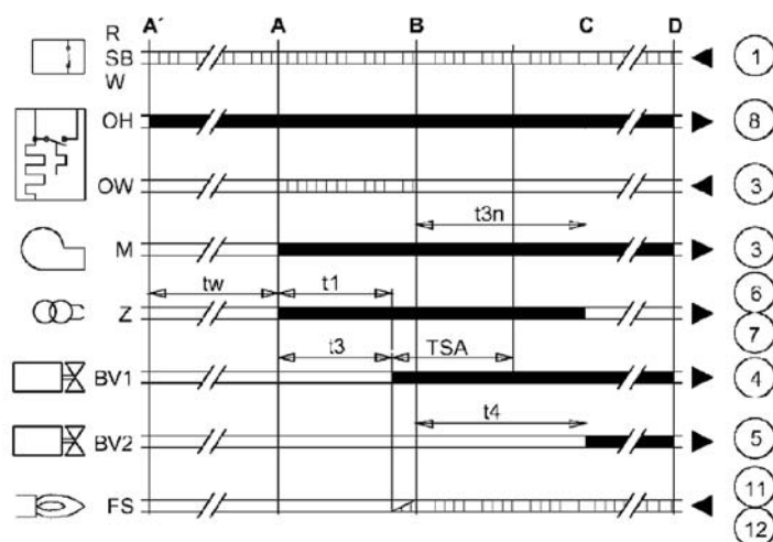
fig. 29 - Ciclo dell'apparecchiatura
