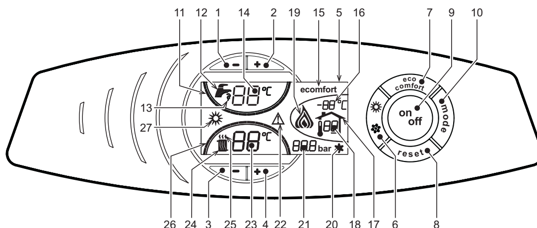
fig. 1 - Pannello di controllo
