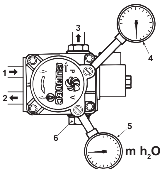
fig. 24 - Pompa
